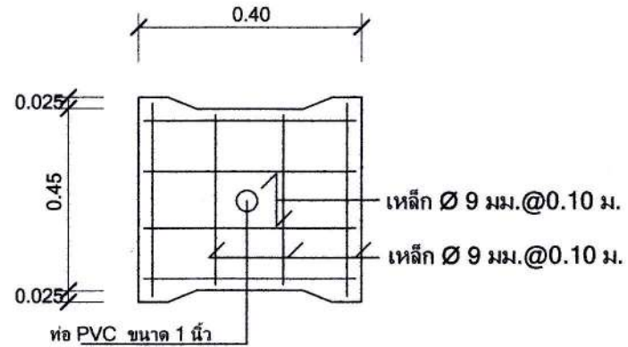
ฝารางระบายน้ำ Not To Scale
