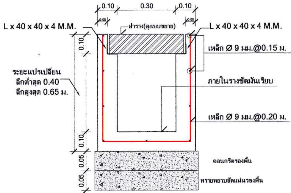
รูปตัดขวางระบายน้ำ Not To Scale
